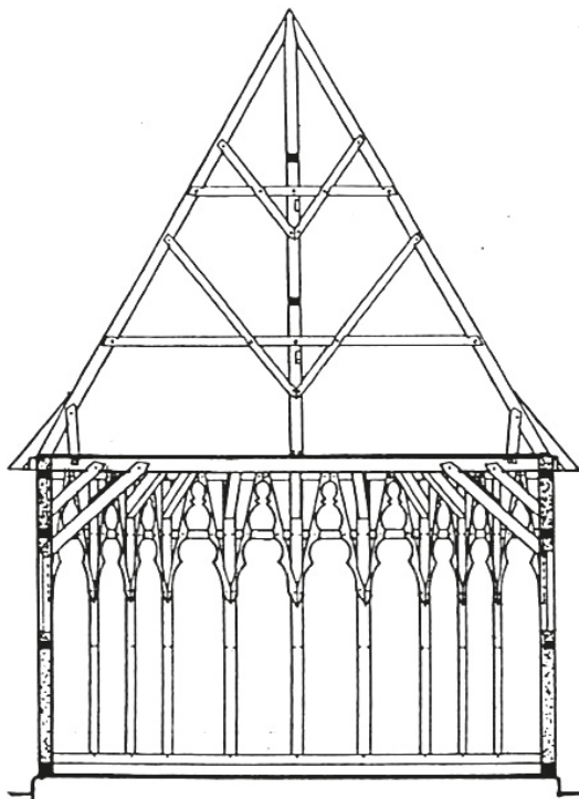
rys. konstrukcji ryglowej wg. prof. J. Tajchmana
